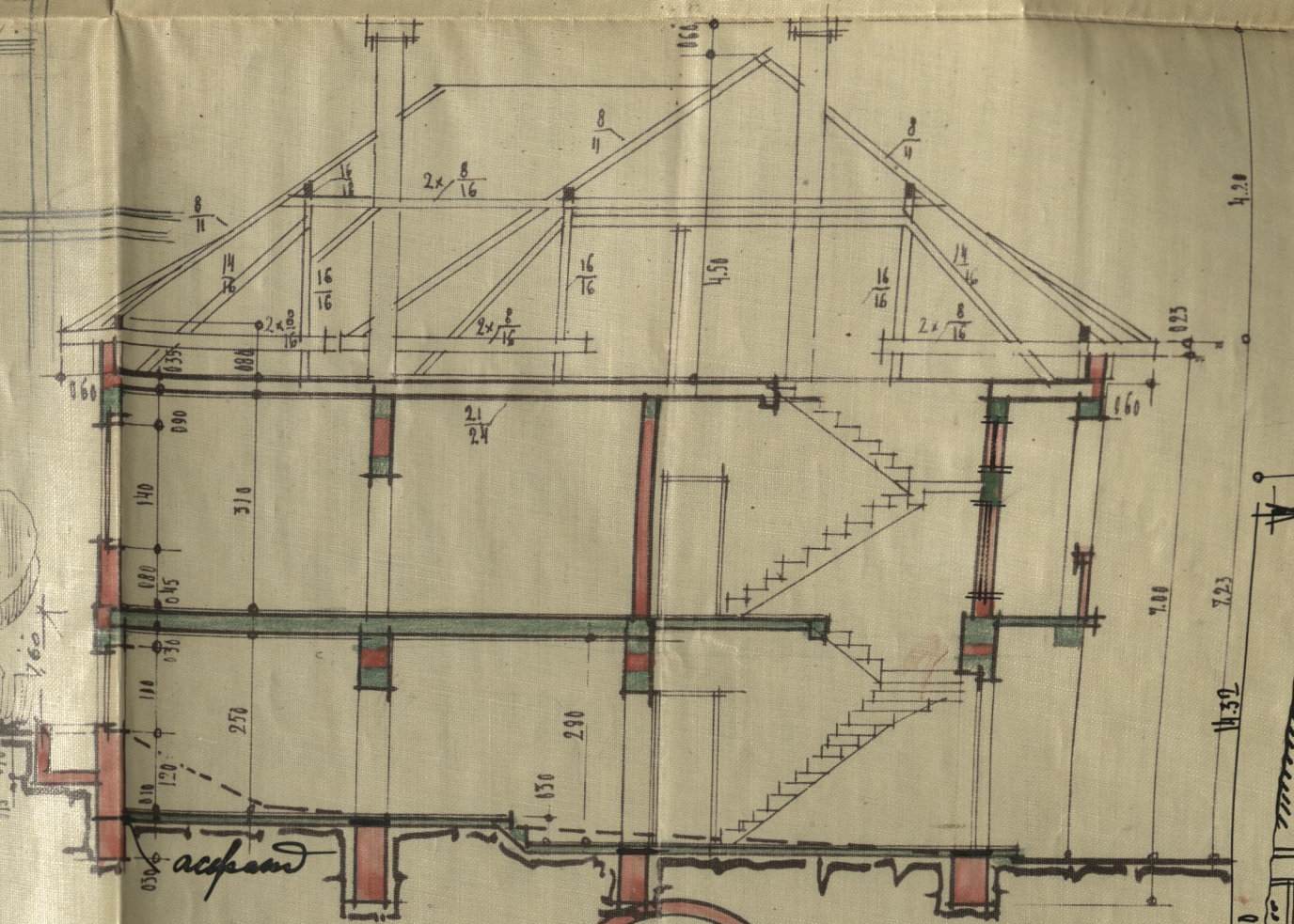
ПРЕСЕК КРОЗ СТЕПЕНИШТА
