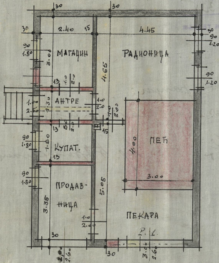
ПРИЗЕМЉЕ
