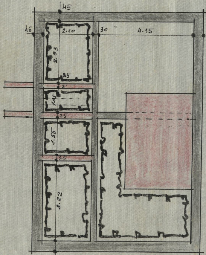
ТЕМЕЉ
