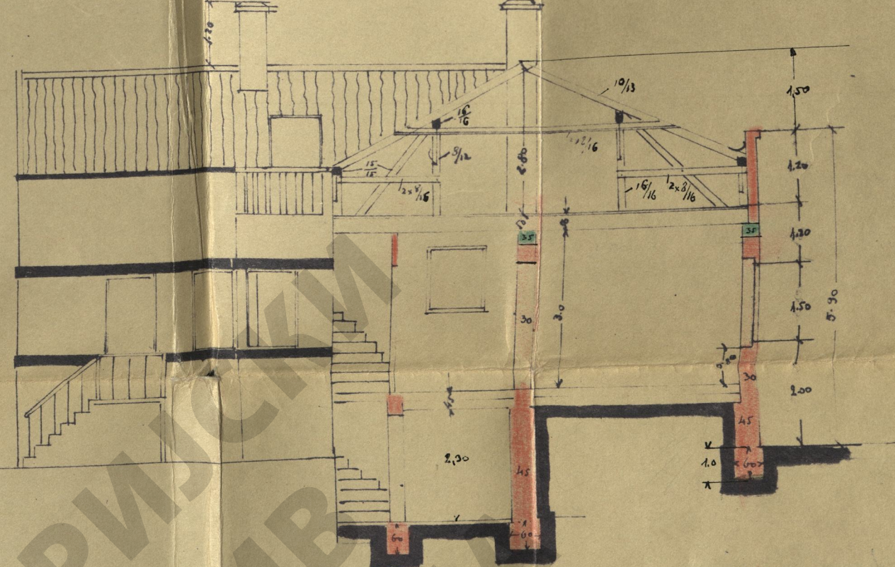
ПРЕСЕК: С-Д
