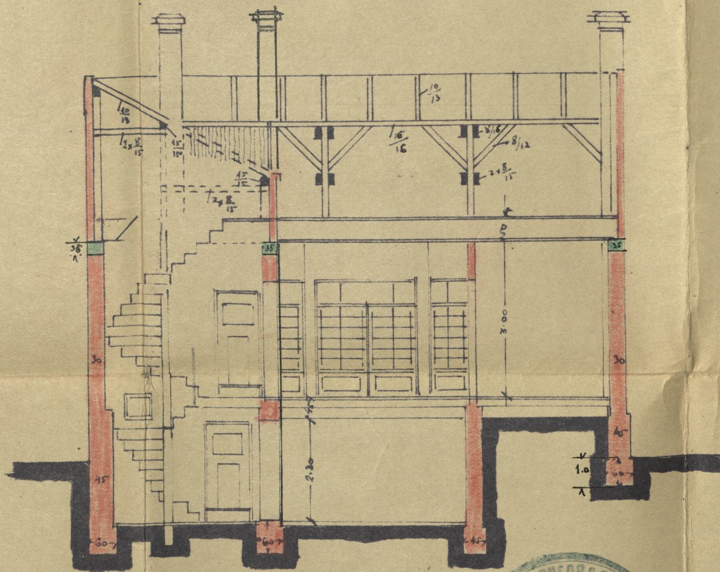
ПРЕСЕК: А-В
