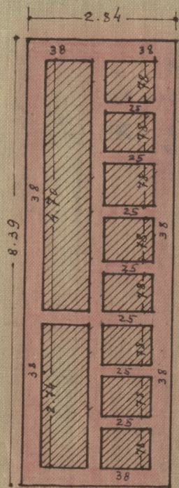
Основа темеља
