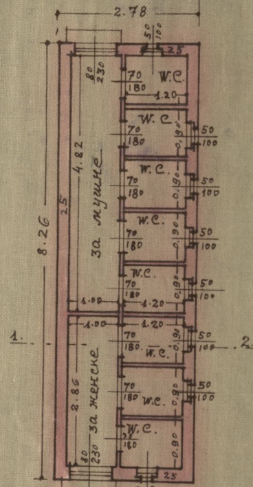
Основа приземља
