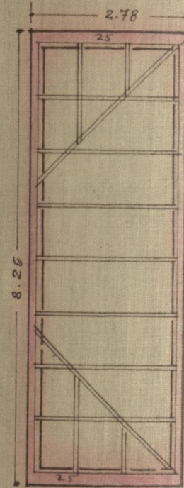
Основа кровља
