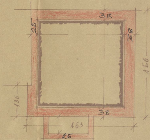
ОСНОВА ТЕМЕЛА
