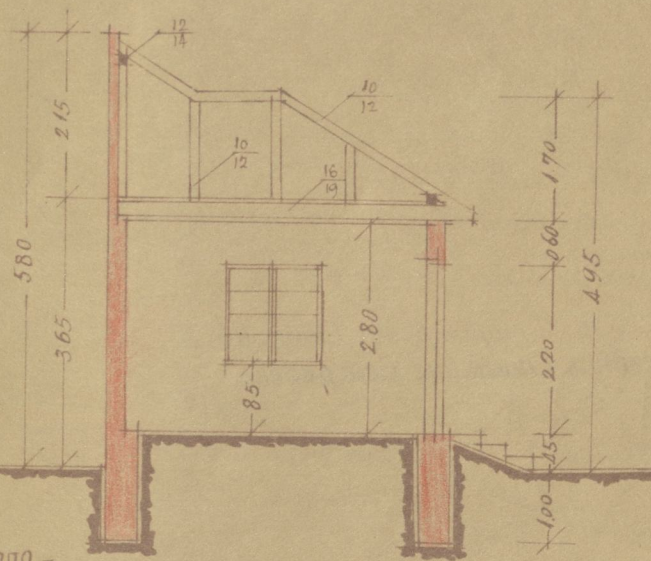
ПРЕСЕК А-Б
