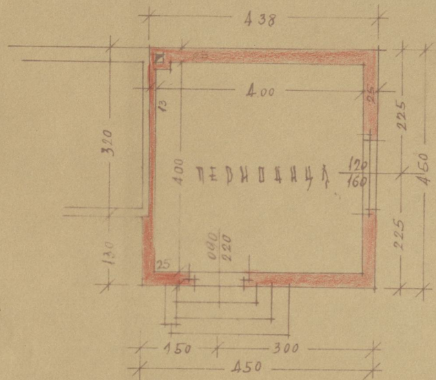
ОСНОВА ПРИЗЕМА
