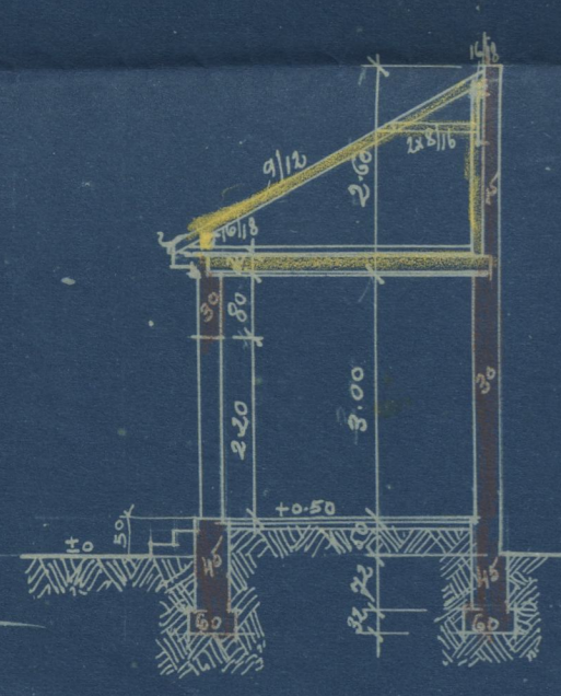
Пресек С-Д.
