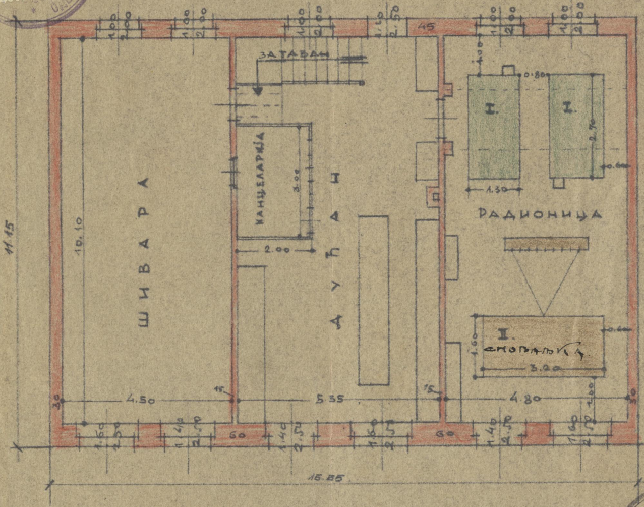
ОСНОВА ПРИЗЕМЉА 1:100
