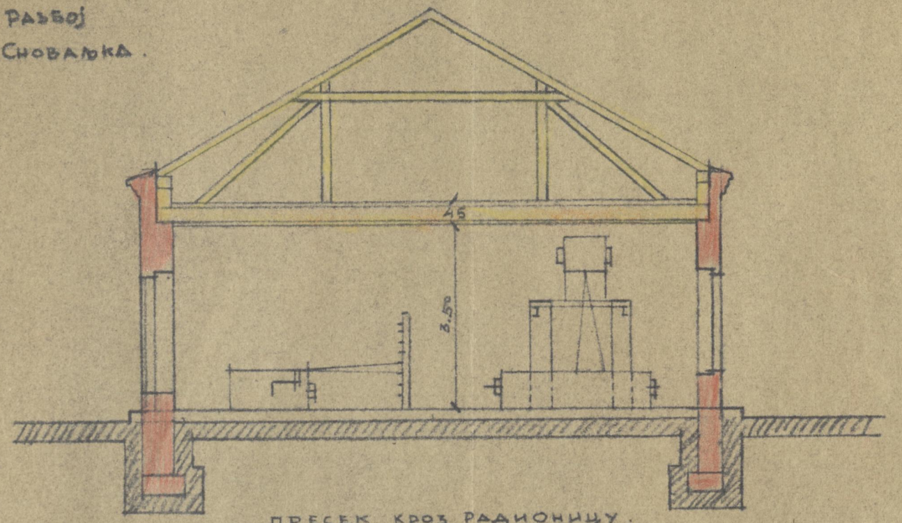
ПРЕСЕК КРОЗ РАДИОНИЦУ 1:100
